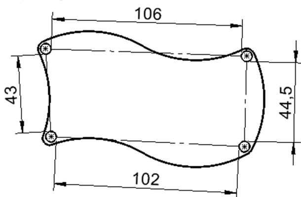
Tischbein-Lichten und Grundmaße (Angaben in [cm])
